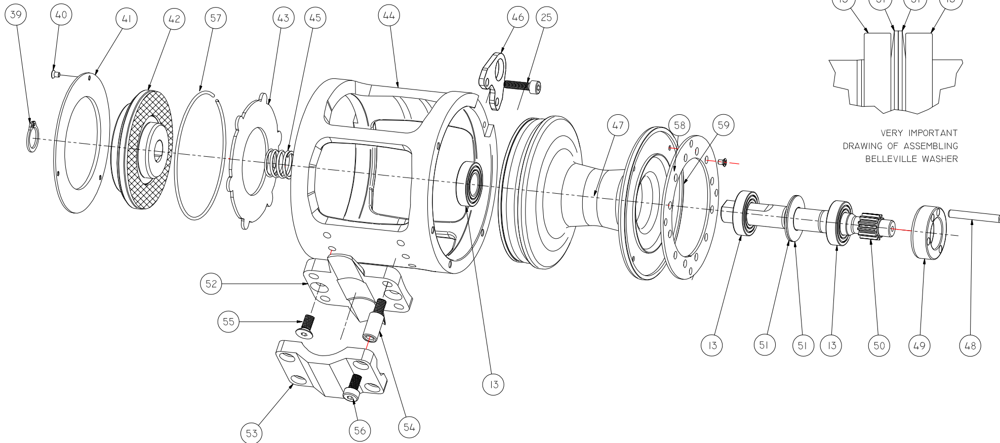
DETTAGLIO POSIZIONAMENTO MOLLE A TAZZA
